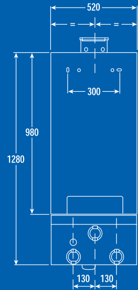
Logamax plus GB162
